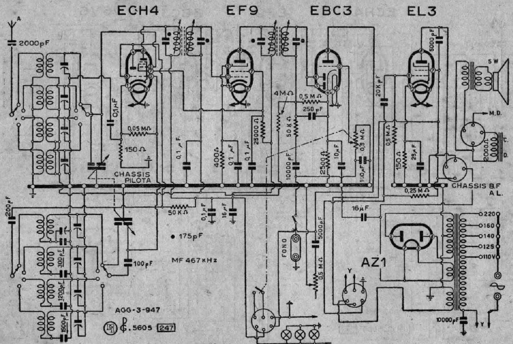
Lo schema elettrico del mod. 542 R
